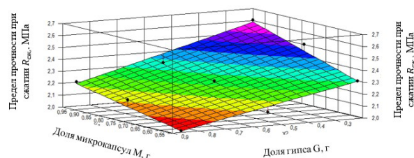
Рис. 4. Зависимость предела прочности на сжатие R_{сж} от доли микрокапсул M и доли гипса G
