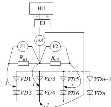
Рис. 7. Устройство диагностирования СПП в преобразователе без резисторов связи
