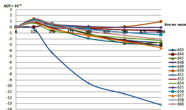
Рис. 7. График зависимости относительного ухода частоты от времени
