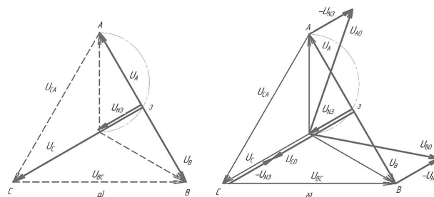
Рис. 2. Векторные диаграммы при R_{\text{гг}} = R_{\text{гг}2} для фазных напряжений (а) и напряжений по уравнению (3) (б)
