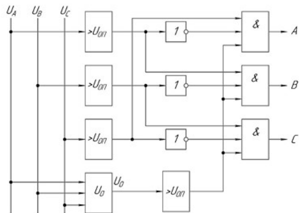
Рис. 4. Структурная схема ИПФ с объединением двух алгоритмов
