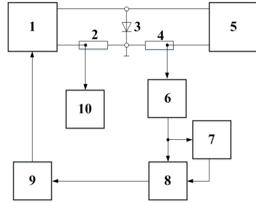
Рис. 1. Блок-схема устройства для измерения величины ударного тока силовых полупроводниковых приборов
