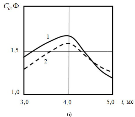
Рис. 2. Вольт-амперные характеристики (а) и зависимости динамической емкости от времени (б) для тиристора Т-25 при высоких плотностях тока, где 1 — расчетные кривые, 2 — экспериментальные кривые
