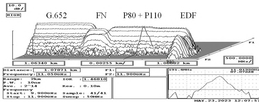
Рис. 6. 3D-BOTDR-рефлектограмма CPMB для световода с эрбиевым ОВ на конце
