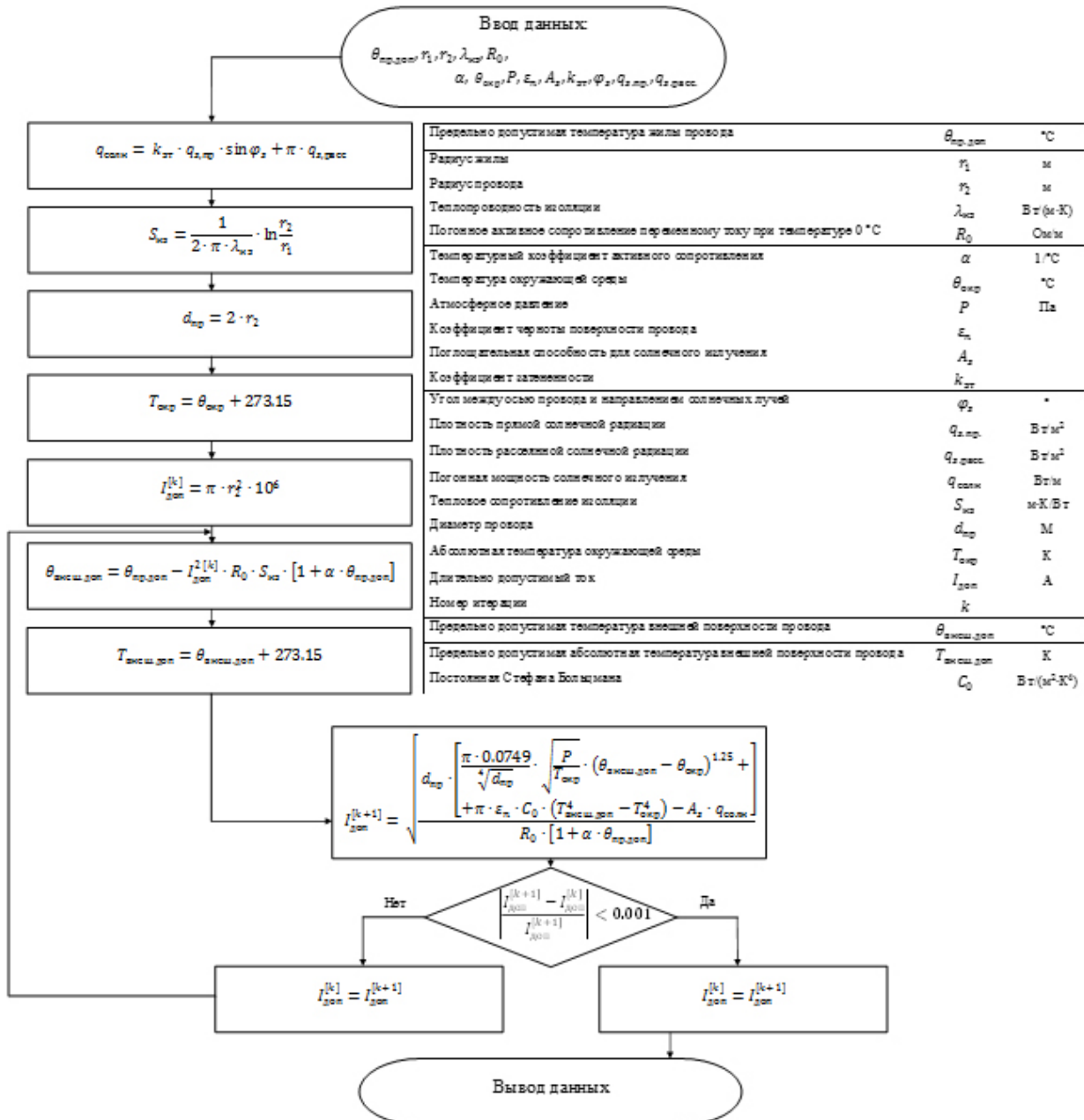
Рис. 1. Алгоритм расчета длительно допустимого тока для естественной конвекции
