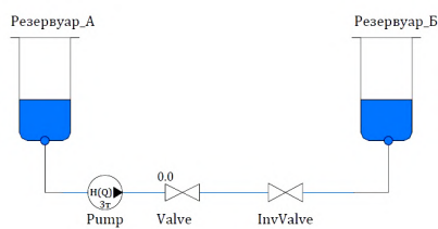
Рис. 2. Гидравлическая подсистема
