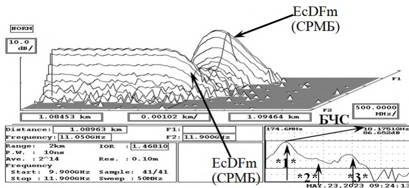
Рис. 3. 3D-BOTDR-рефлектограмма при малой концентрации церия в OB-EcDF (EcDFm)
