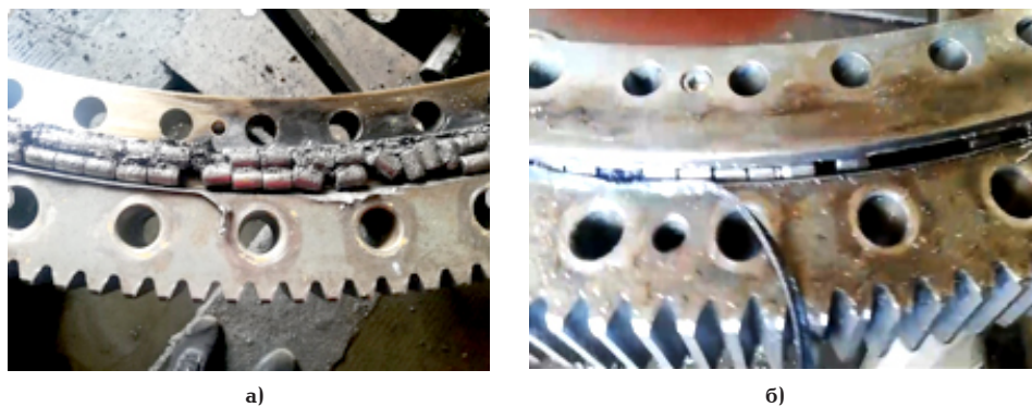
Рис. 1. Характерные отказы ОПУ: а — выпадение тел качения из кассет (сепараторов); б — выдавливание уплотнительной ленты
